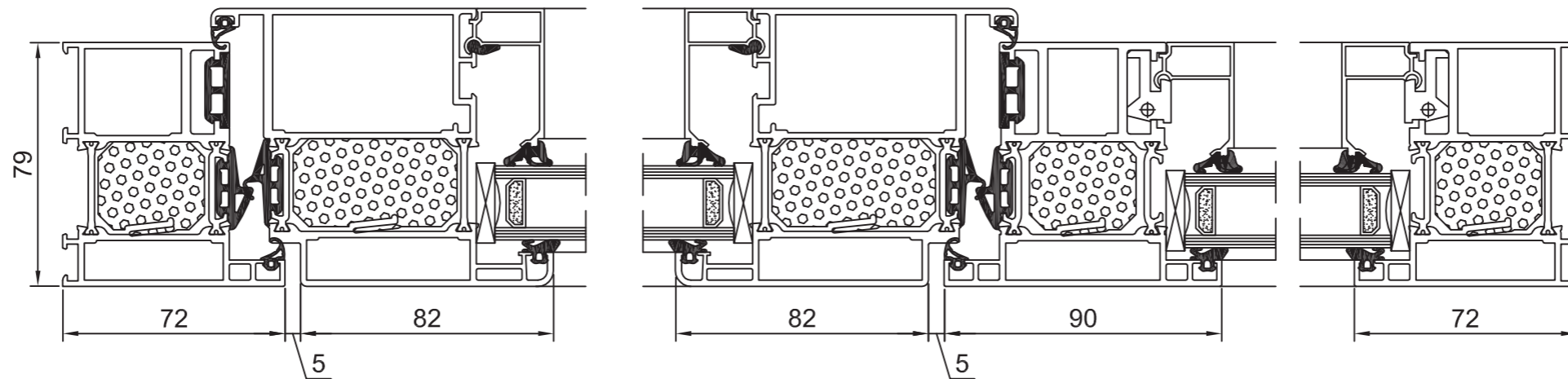
ARCADE Elementbauweise (Metallbauvariante)
