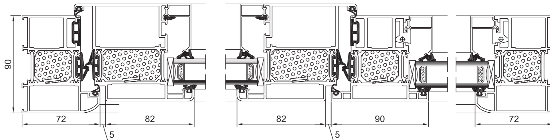
SYMPHONIE Elementbauweise (Metallbauvariante)
